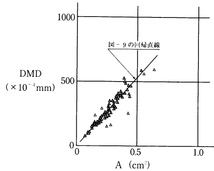
図-10 AとDMDの関係 (実測値)
