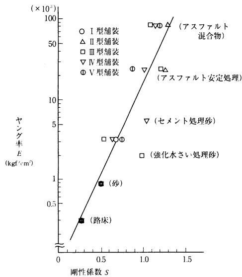
図-4 剛性係数とヤング率の関係
