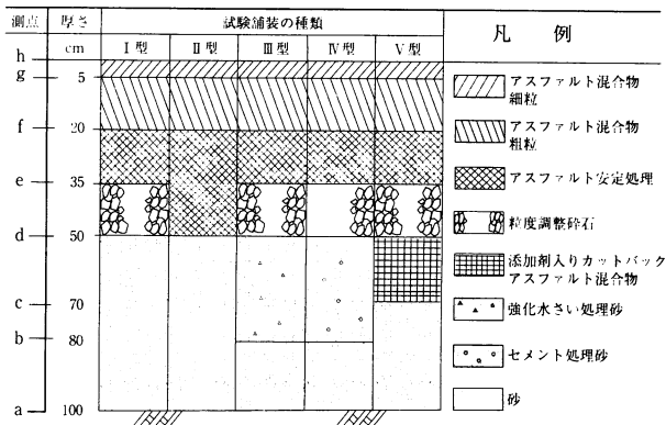
図-3 試験舗装の構造
