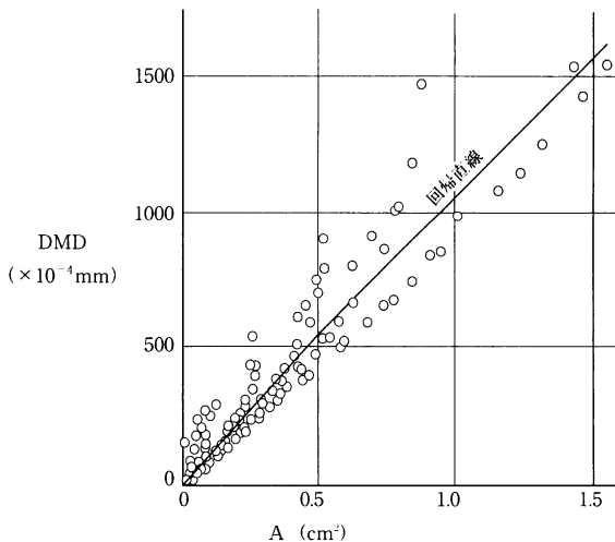
図-9 AとDMDの関係 (理論値)
