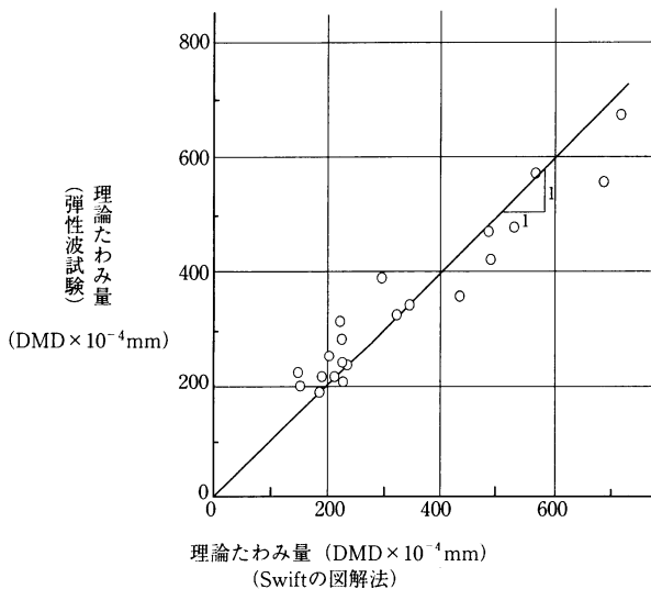
図-7 理論たわみ量の比較
