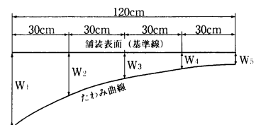
図-8 ダイナフレクトの測定位置
