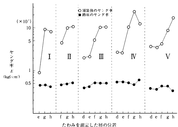
図-5 Swiftの図解法より求めたヤング率
